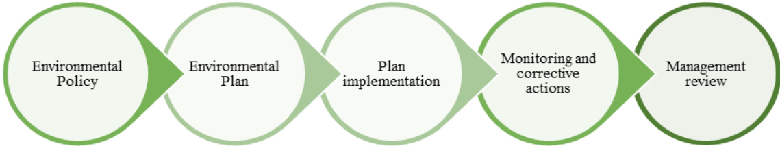
Fig. 1. ISO 14001 diagram
